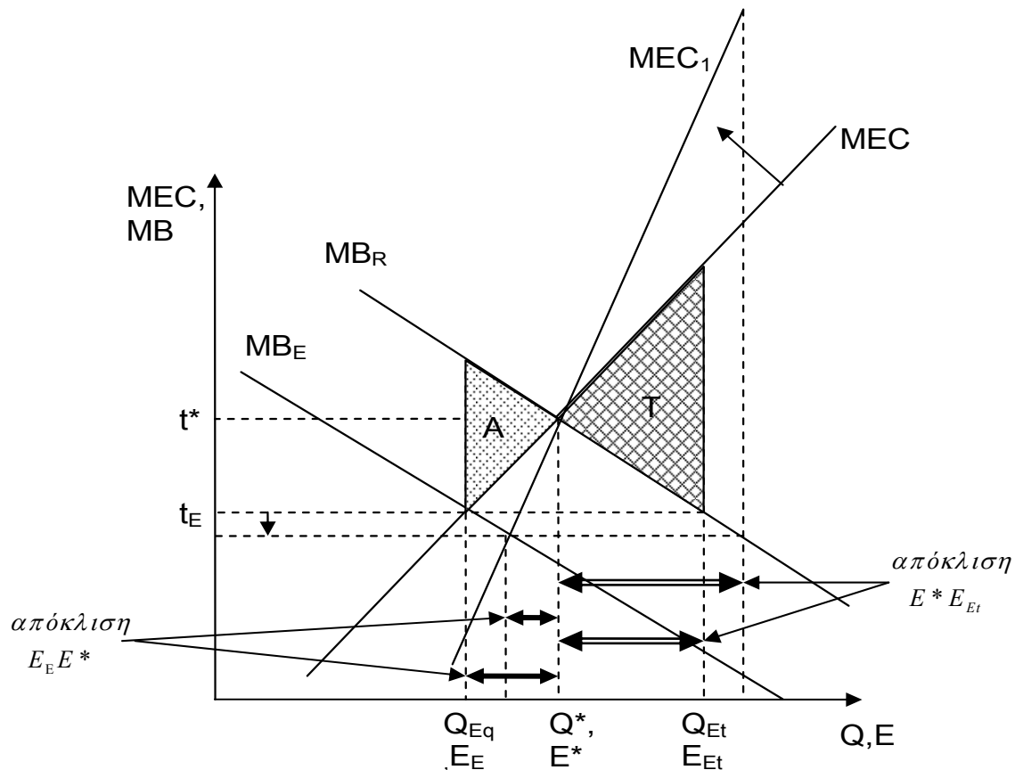
Διάγραμμα 3: Η κλίση της MEC και το μέγεθος της απώλειας κοινωνικής ευημερίας
