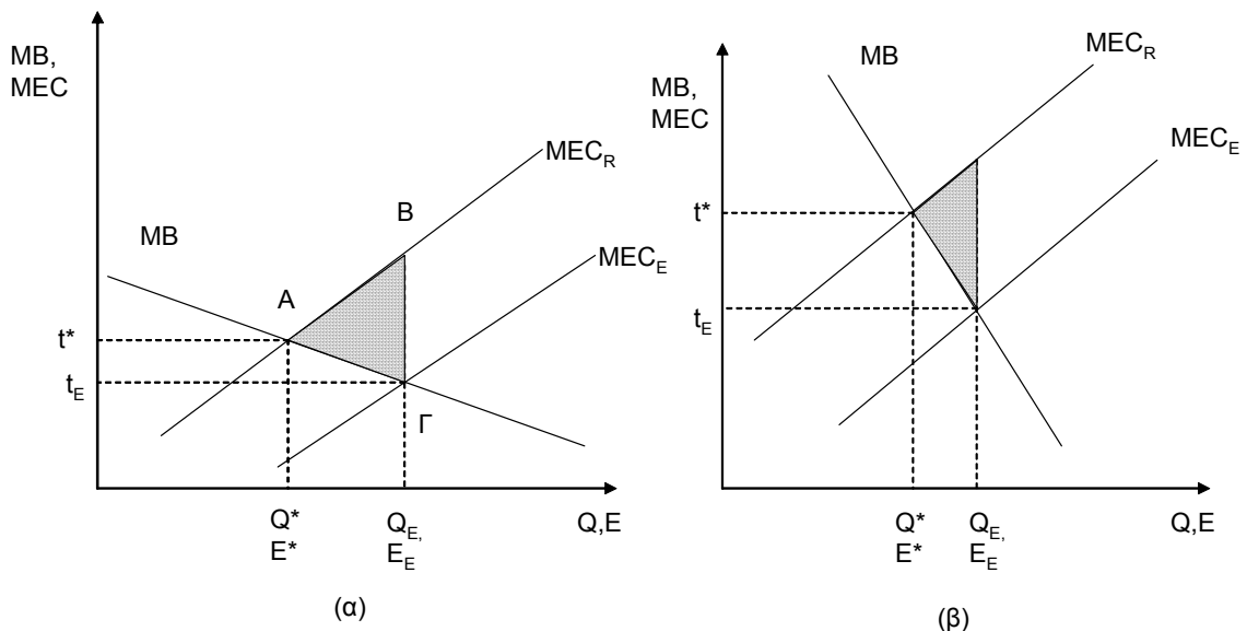
Διάγραμμα 1: Σύγκριση ανώτατων ορίων και φορολογίας όταν επικρατεί αβεβαιότητα σχετικά με την καμπύλη MEC .
