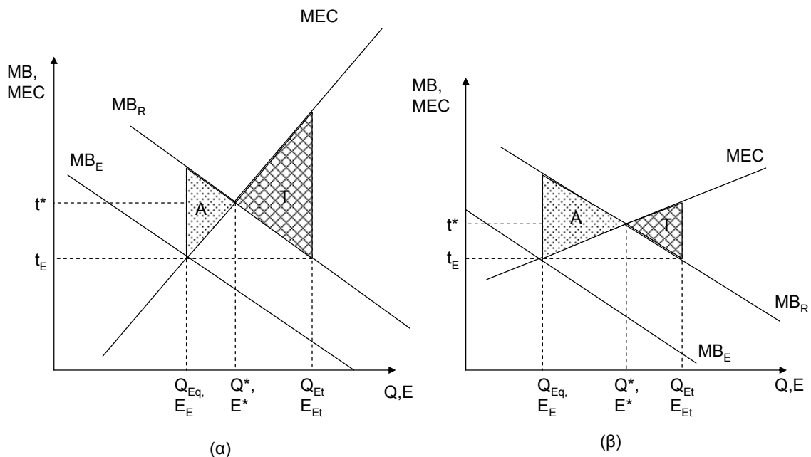
Διάγραμμα 2: Σύγκριση ανώτατων ορίων και φορολογίας όταν επιρρατεί αβεβαιότητα σχετικά με την καμπύλη MB
