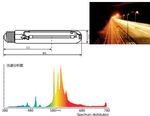
Λάμπες Νατρίου
